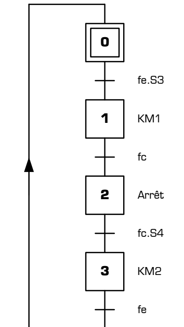
Exemple de grafcet du point de vue « partie commande »
