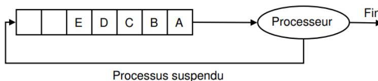
Ordonnancement circulaire
