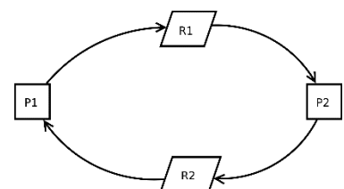
Exemple d'interblocage :
